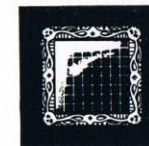
Blip tokens
